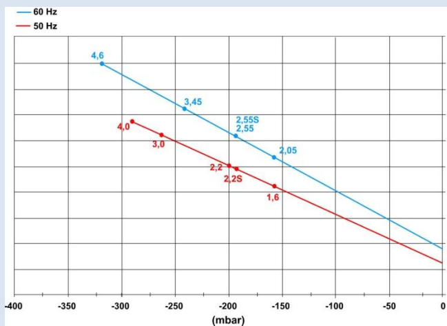
Potencia requerida en el eje de la soplante / Power requirement on the blower shaft
