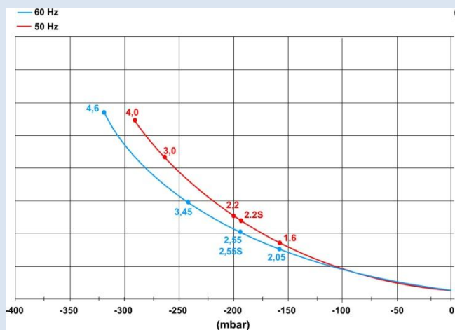
Aumento de la temperatura del aire vehiculado / Temperature rise on the exhaust air
