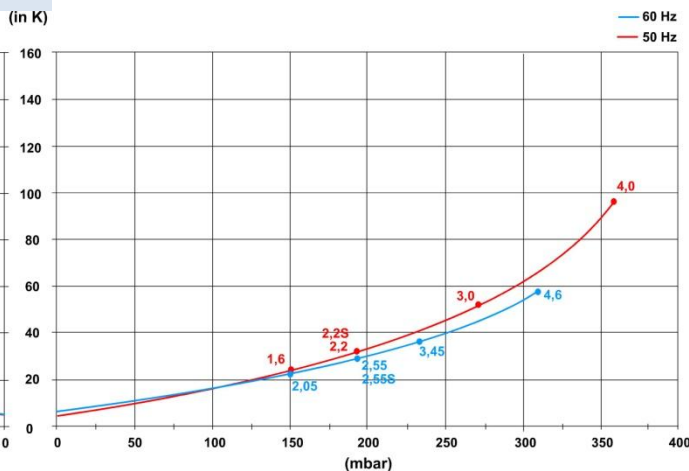
Aumento de la temperatura del aire vehiculado / Temperature rise on the exhaust air
